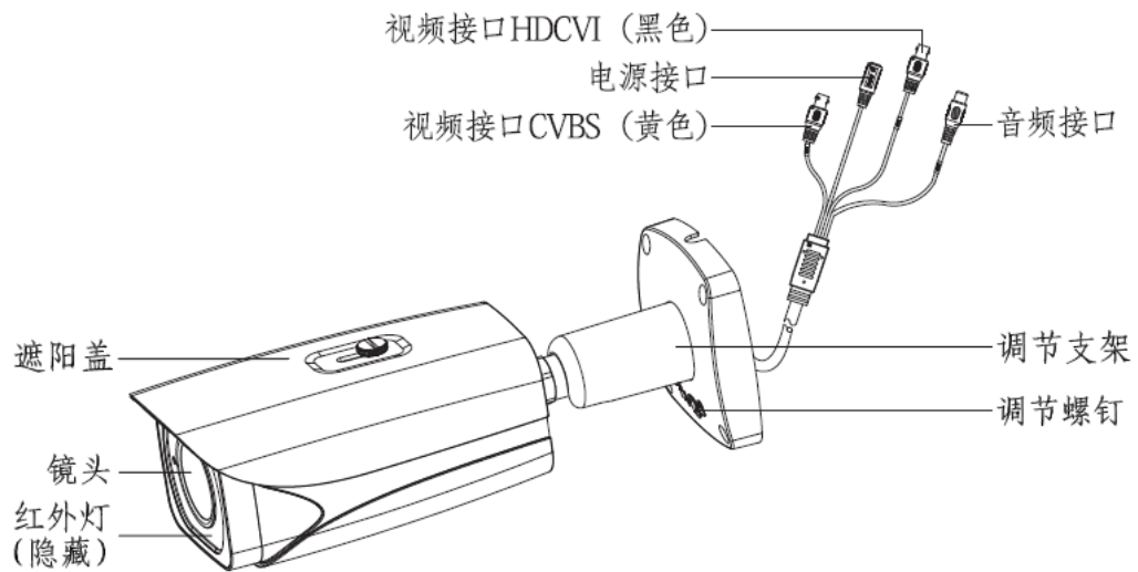
图2-8 优雅型电动变焦红外防水枪机 DH-HAC-HFWXXXXE-Z 型结构部件图（2）
