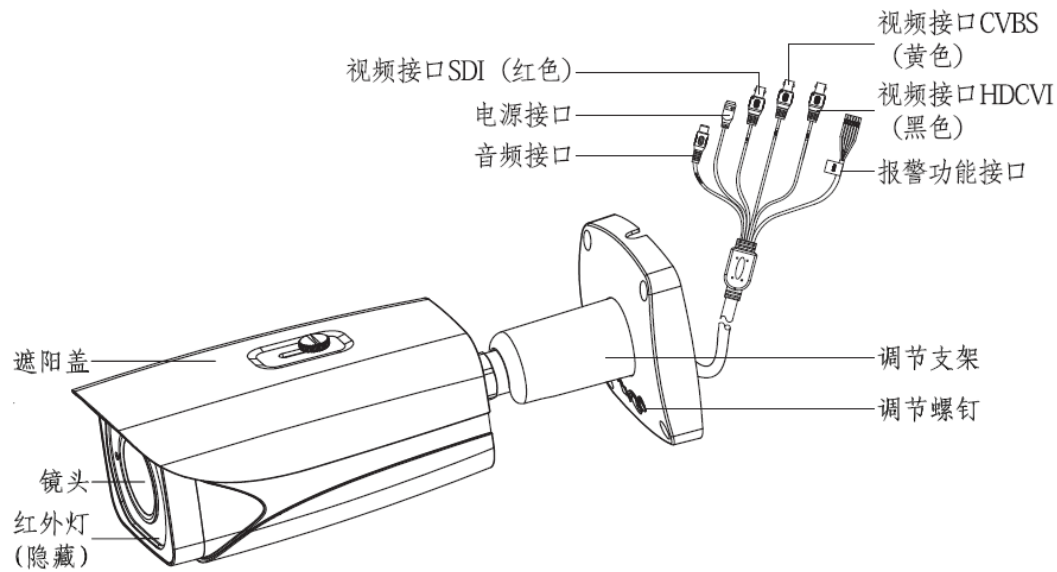
图2-9 优雅型全功能电动变焦红外防水枪机 DH-HAC-HFWXXXXE-Z 型结构部件图（1）
