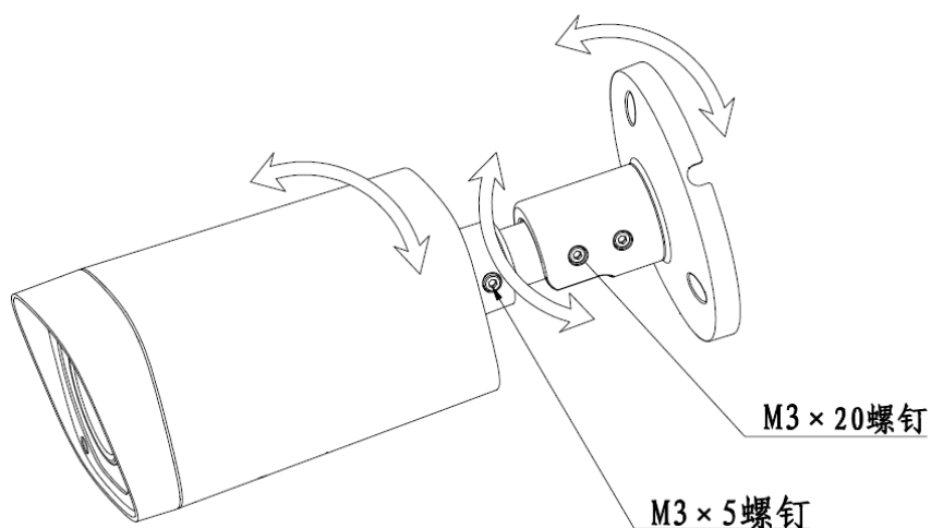
图3-3 安装示意图（3）
