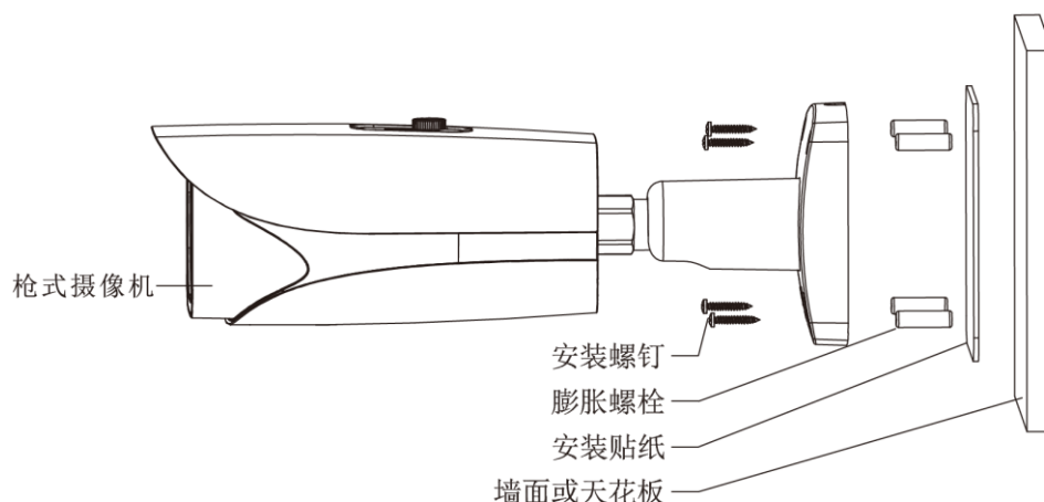
图3-1 安装示意图（1）
