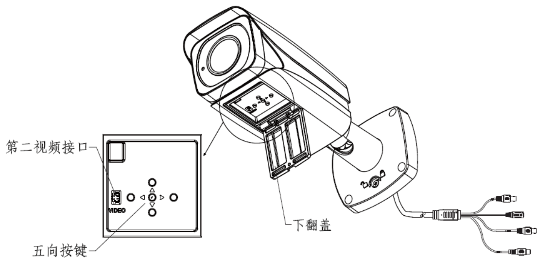
图2-8 优雅型电动变焦红外防水枪机 DH-HAC-HFWXXXXE-Z 型结构部件图（2）
