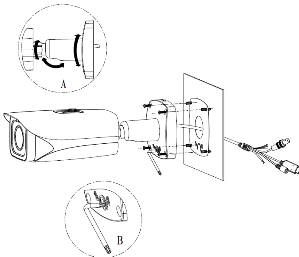
图3-2 安装示意图（2）
