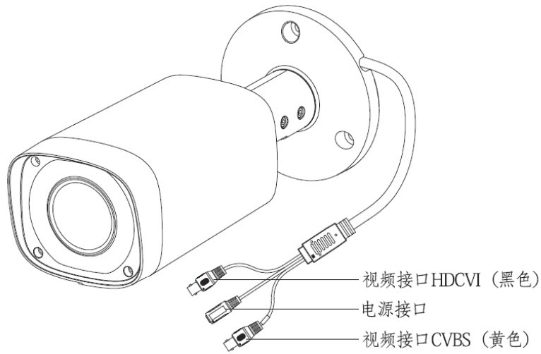
图2-4 电动变焦红外防水枪机 DH-HAC-HFWXXXXR-Z 型/手动变焦红外防水枪机 DH-HAC-HFWXXXXR-VF 型结构部件图
