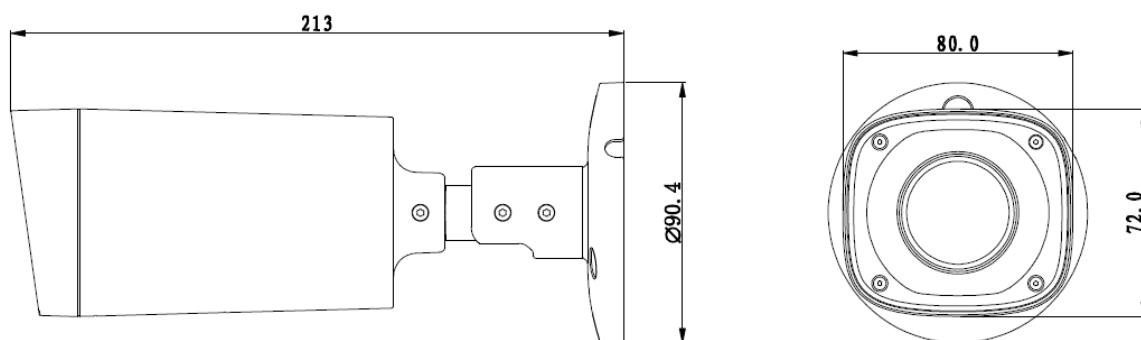
图2-2 手动变焦红外防水枪机 DH-HAC-HFWXXXXR-VF 型结构尺寸图（单位：mm）
