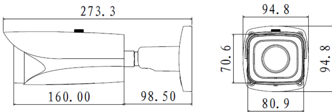
图2-3 优雅型电动变焦红外防水枪机 DH-HAC-HFWXXXXE-Z 型/DH-HAC-HFWXXXXE-SD 型 /DH-HAC-HFWXXXXE-SVF 型结构尺寸图（单位：mm）
