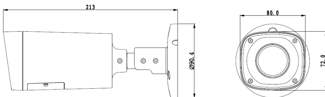
图2-3 优雅型电动变焦红外防水枪机 DH-HAC-HFWXXXXE-Z 型/DH-HAC-HFWXXXXE-SD 型 /DH-HAC-HFWXXXXE-SVF 型结构尺寸图（单位：mm）
