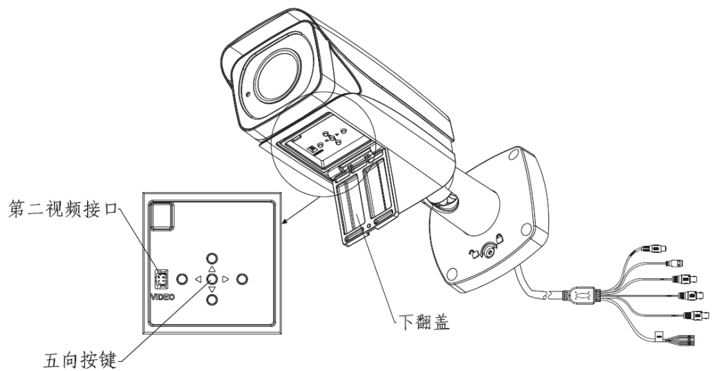
图2-10 优雅型全功能电动变焦红外防水枪机 DH-HAC-HFWXXXXE-Z 型结构部件图（2）
