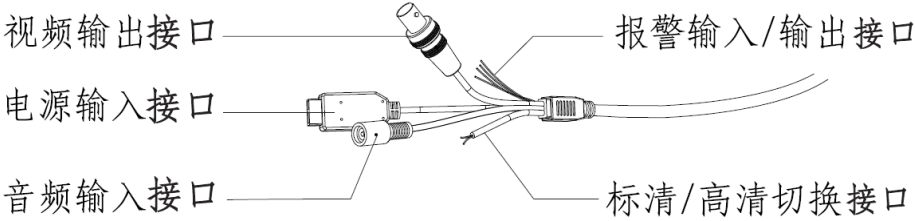
图2-12 结构线缆图（2）
