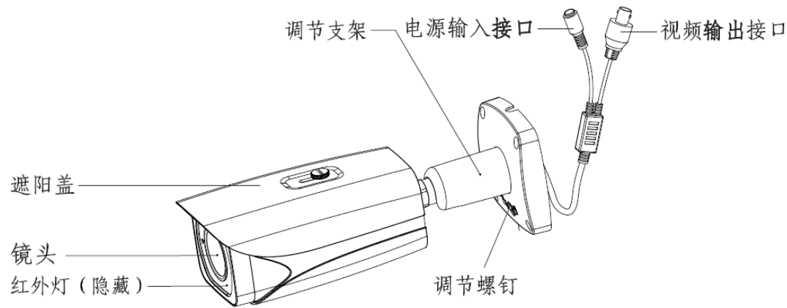
图2-12 结构线缆图（2）
