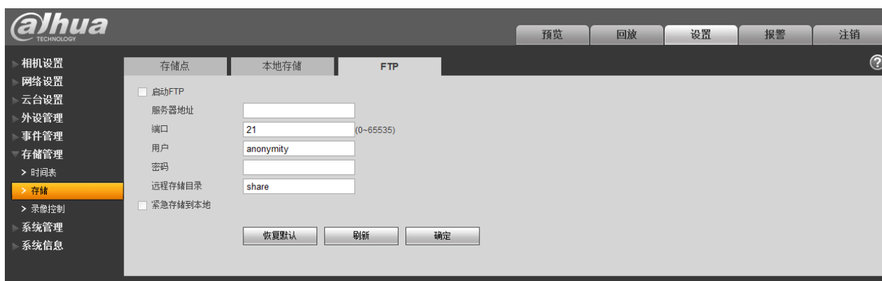
图 3-66 存储管理-FTP 示意图
