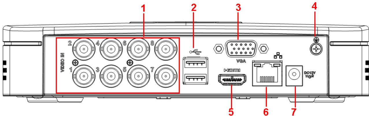
图2-13 2108C-W 系列
