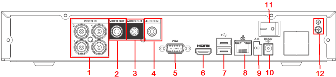
图2-17 5104H 后面板
