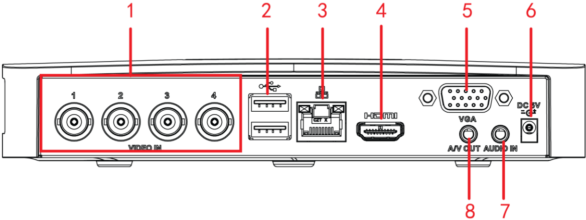
图2-8 DVR504 后面板
