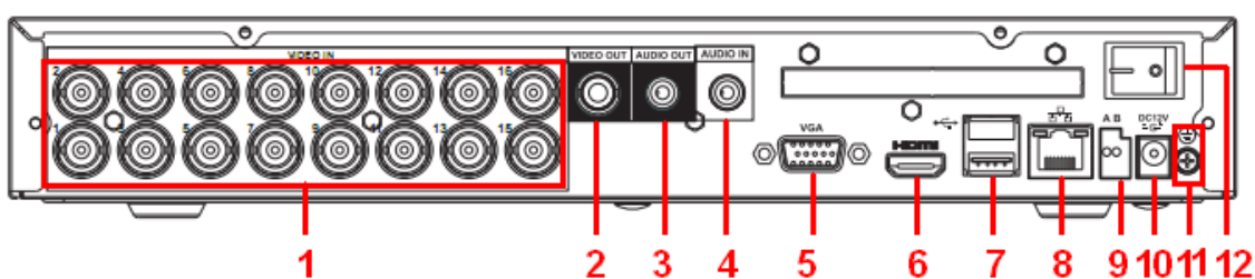
图2-19 5116/2116H 后面板
