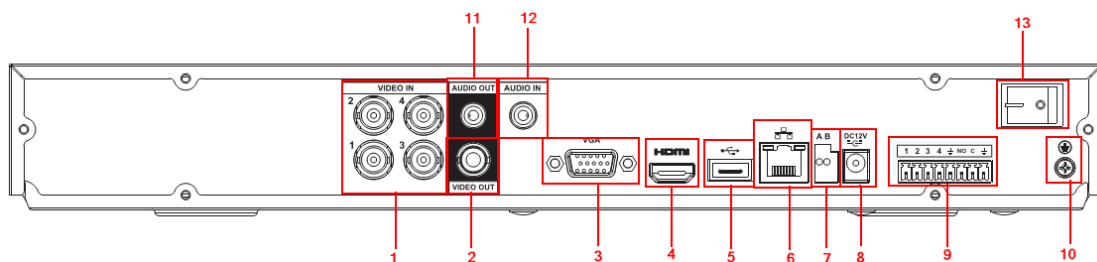
图2-20 5104HE 后面板
