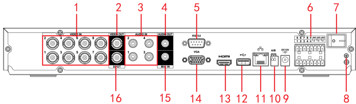
图2-27 DVR2208A 后面板
