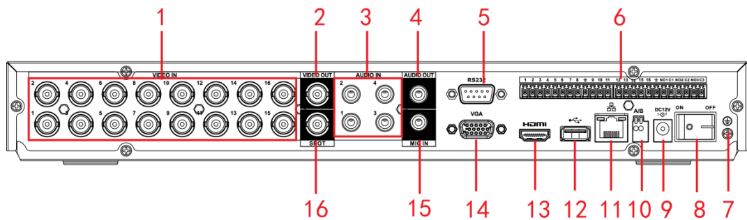
图2-28 DVR2216A 后面板
