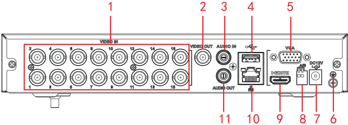
图2-16 2116HS 后面板
