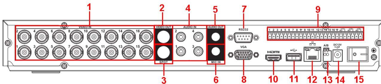
图2-23 52A 系列
