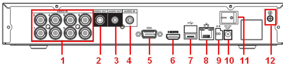
图2-18 5108H 后面板
