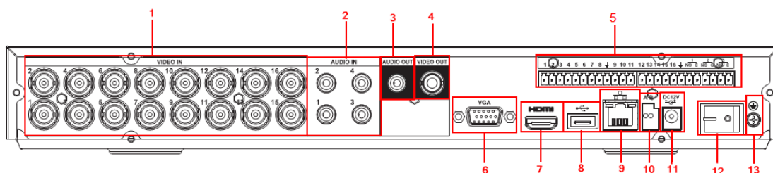
图2-22 5116HE/2116HE 后面板
