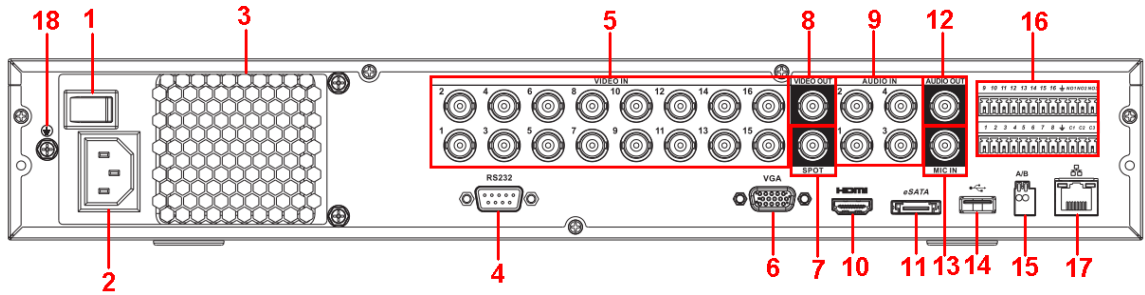
图2-24 5416 后面板
