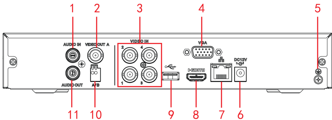
图2-14 2104HS 后面板
