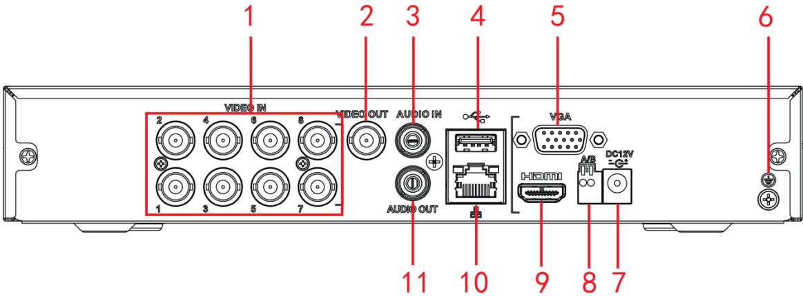
图2-15 2108HS 后面板
