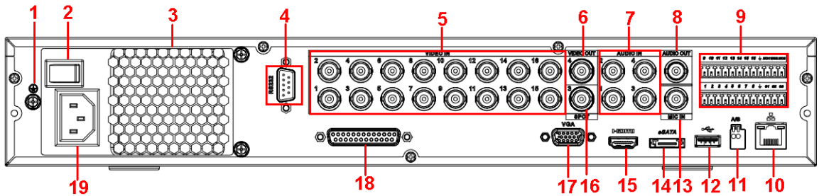
图2-25 5416-L 后面板
