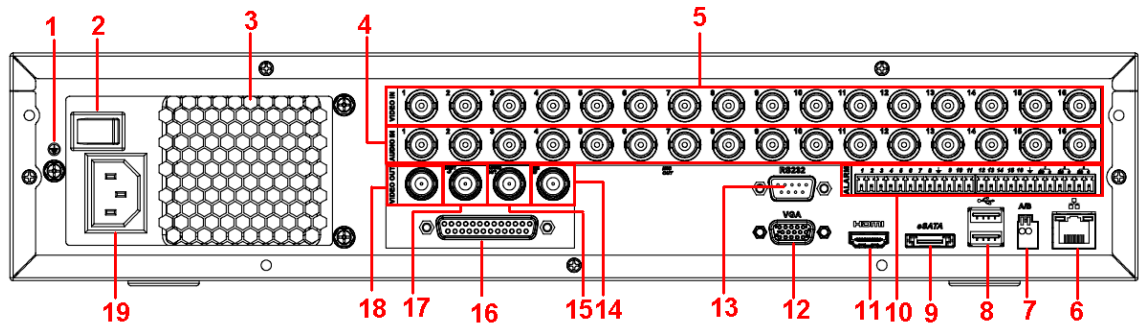
图2-26 5816-S 后面板
