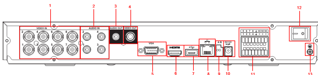
图2-21 5108HE 后面板
