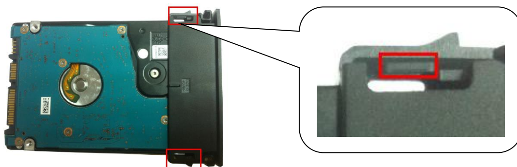
图3-1 拆卸硬盘
