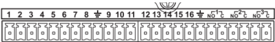
图3-7 DVR52A 系列
