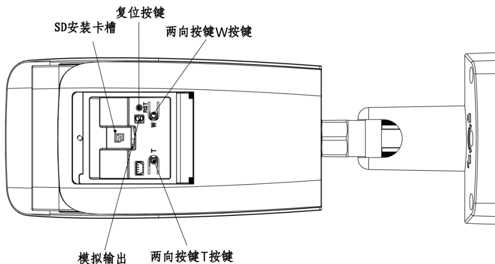
图3-2 SD 卡及按键示意图
