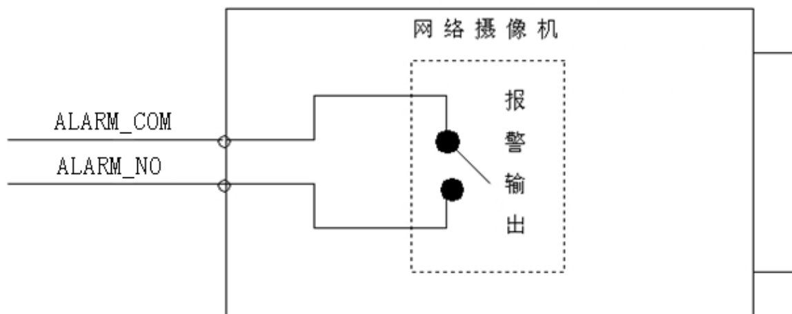
图2-5 报警输出示意图
