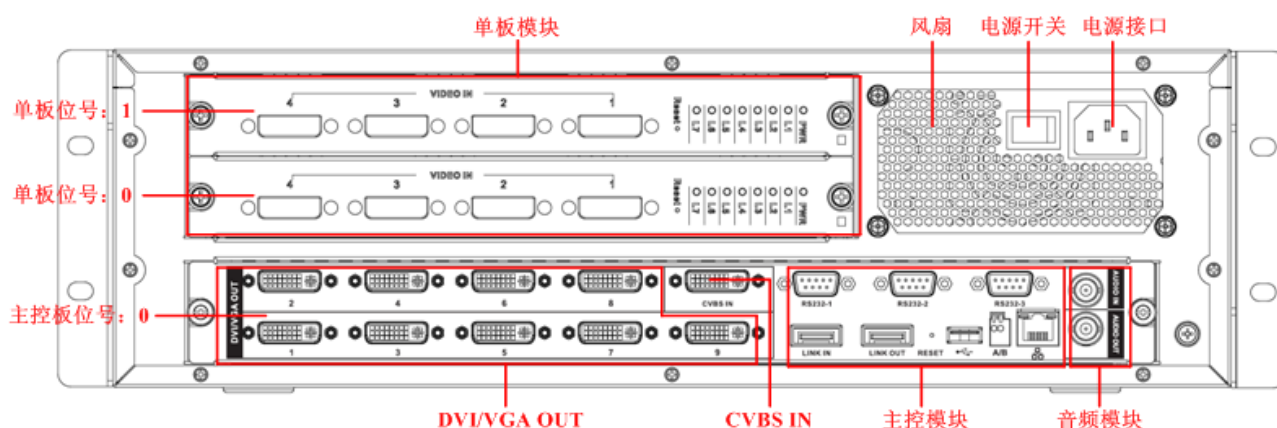
图5-1 后面板
