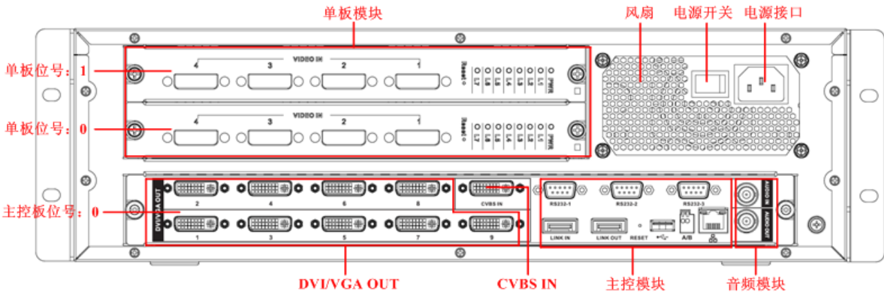
图2-2 DH-M30-3U 后面板
