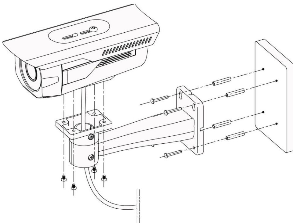
图 3-2 安装示意图
