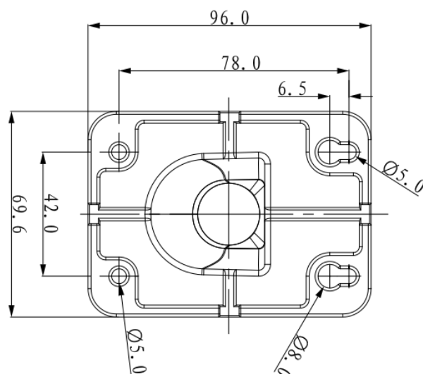
图 3-1 底座孔位图
