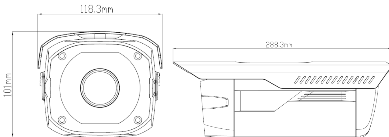
图 7 100 米红外防水枪式摄像机结构尺寸图
