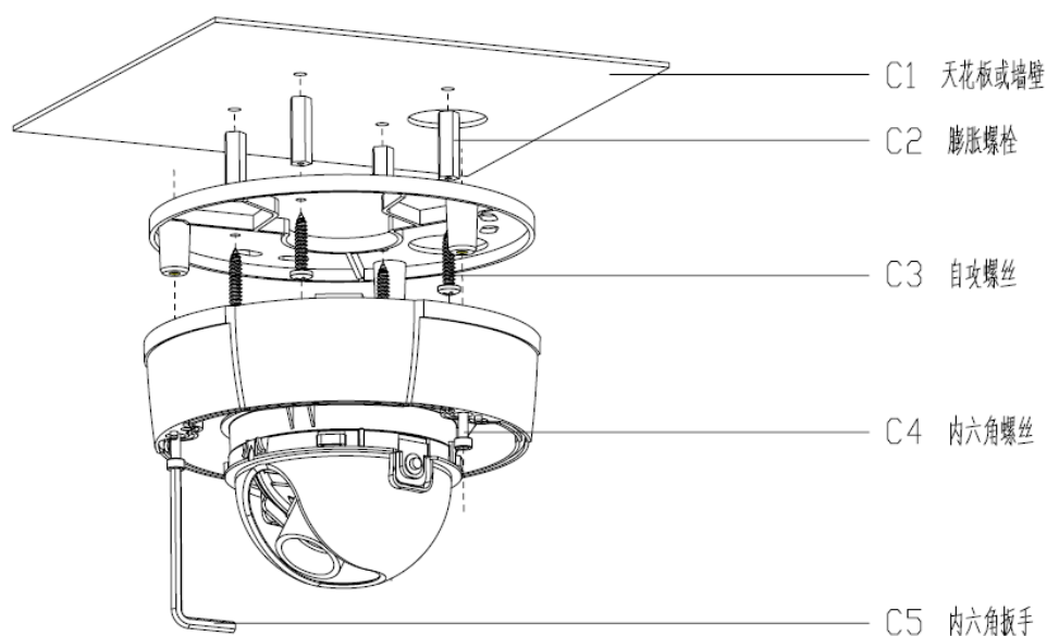
图 25 设备安装示意图（3）
