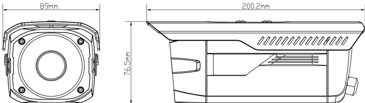
图 6 50 米红外防水枪式摄像机结构尺寸图
