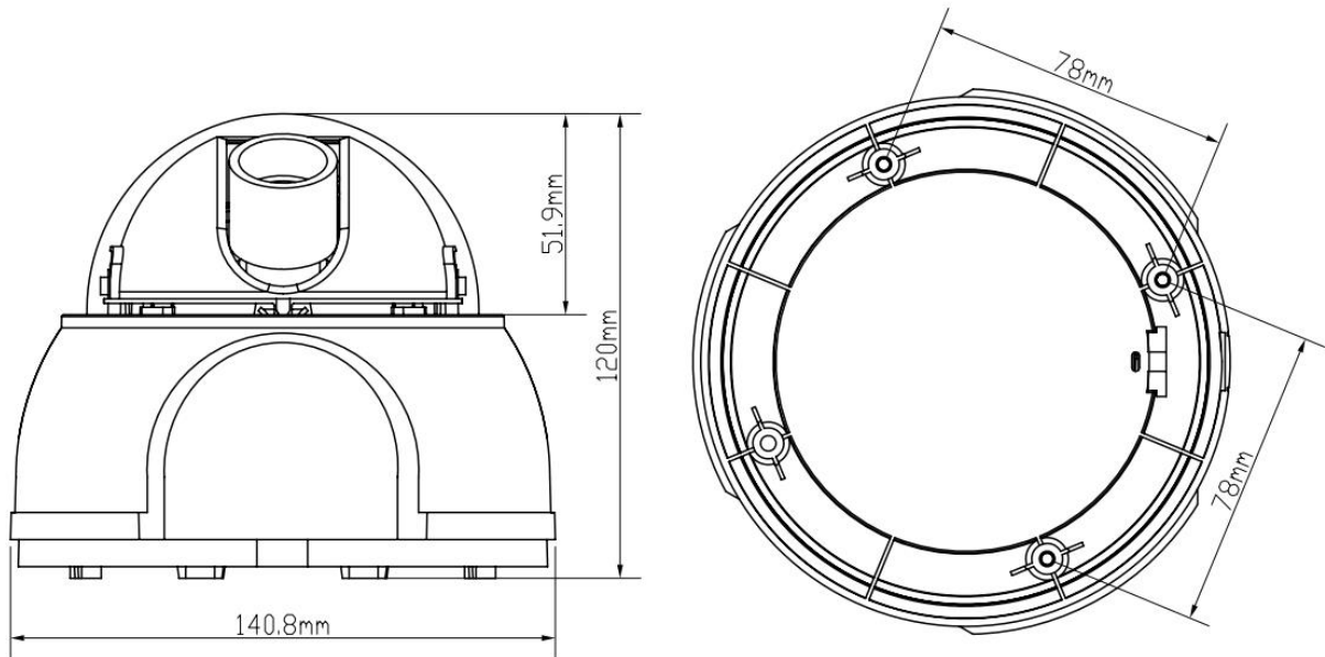
图 5 日夜型超高解像度半球摄像机结构尺寸图
