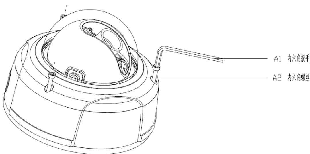
图 23 设备安装示意图（1）
