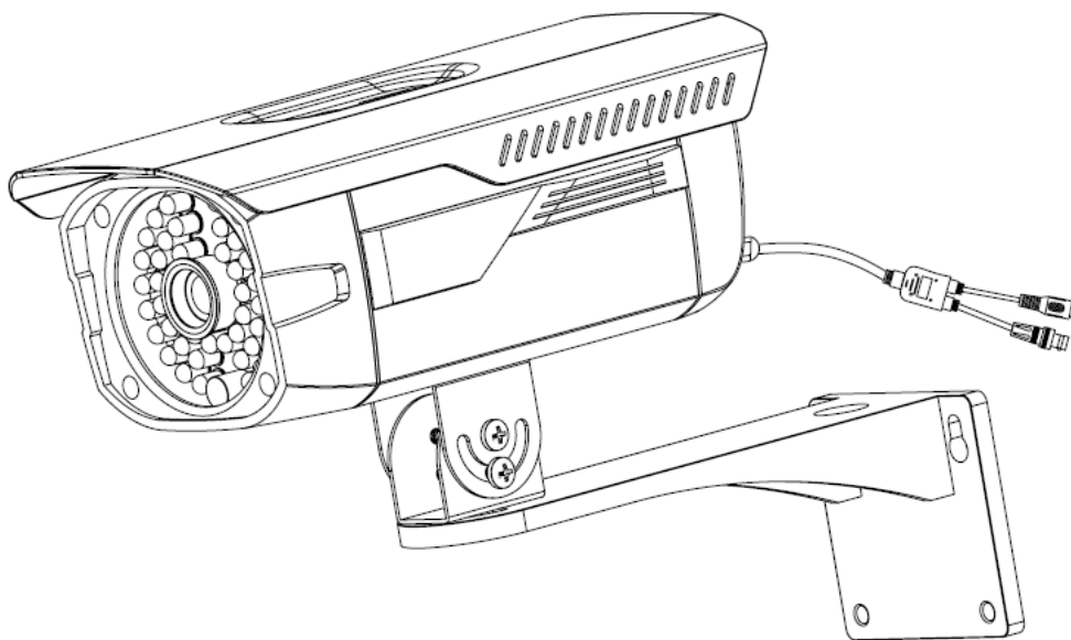
图 3-1 枪机安装示意图
