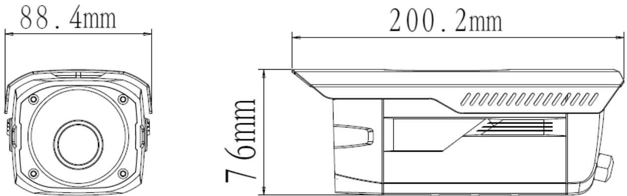
图 2-2 尺寸示意图
