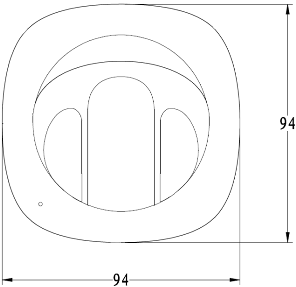
图2-3 结构尺寸示意图（2）（单位：mm）
