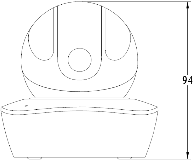
图2-3 结构尺寸示意图（2）（单位：mm）
