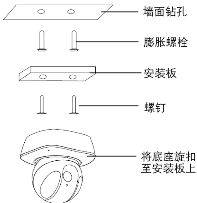
图3-1 安装示意图
